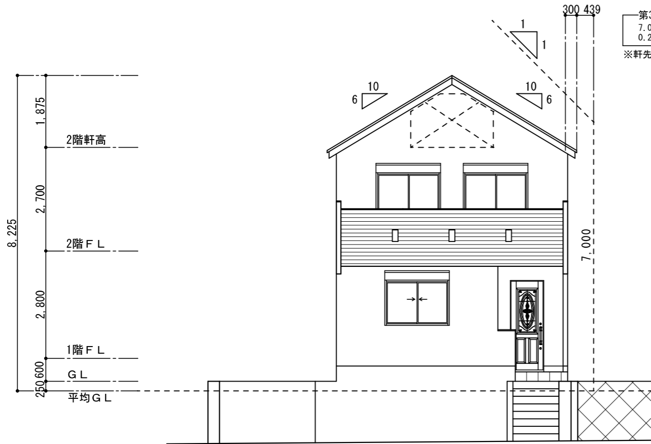
南立面図
