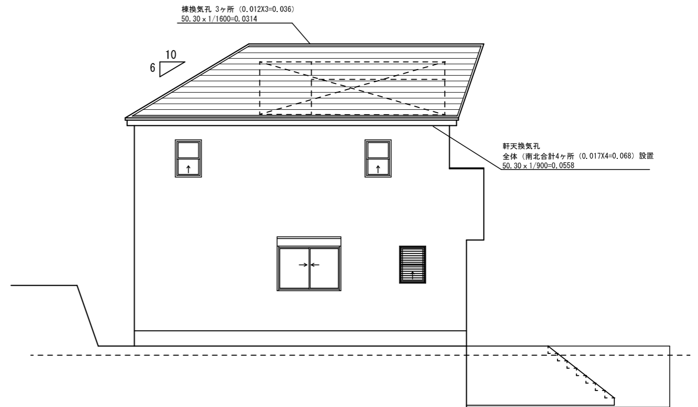
西立面図
