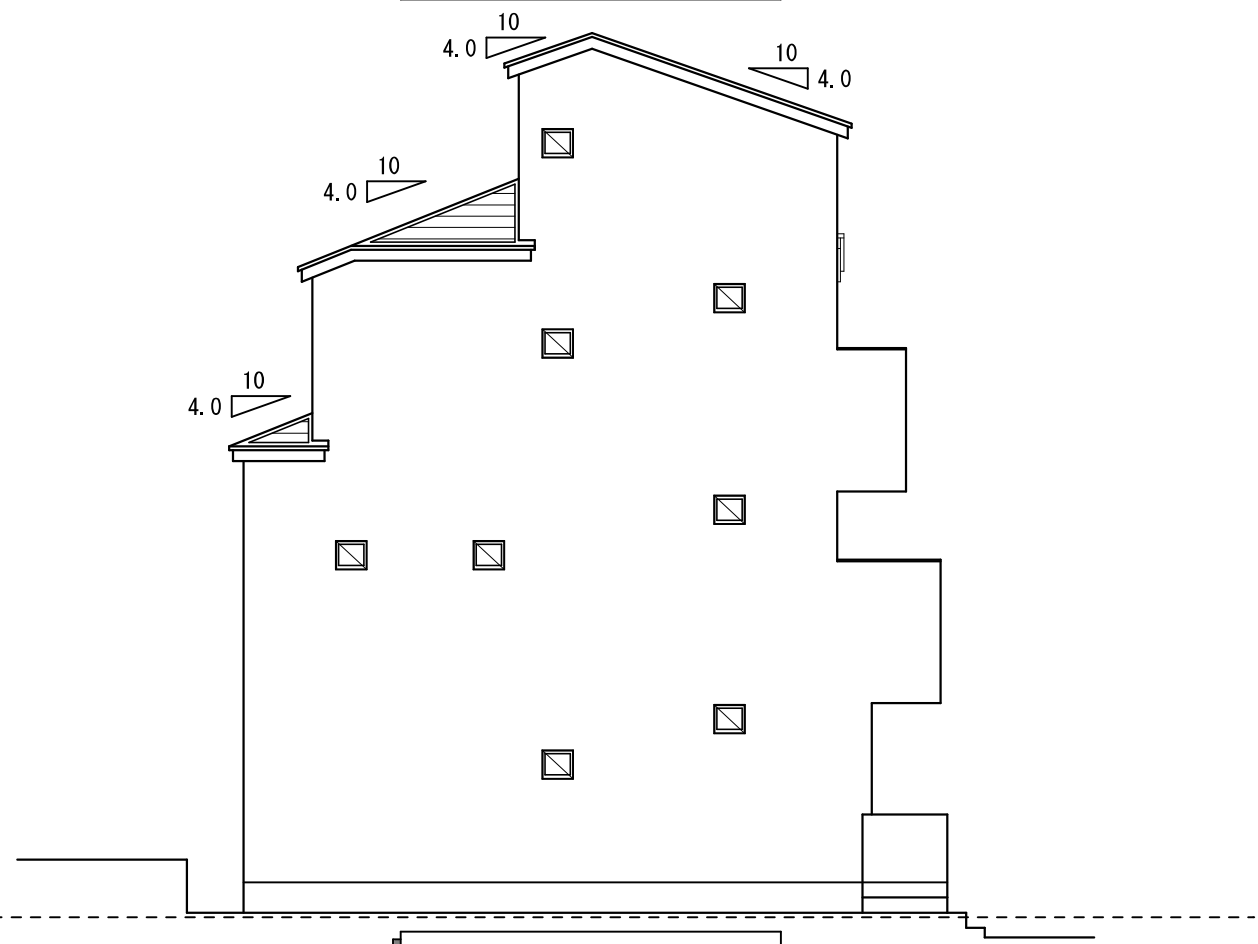
西立面图
