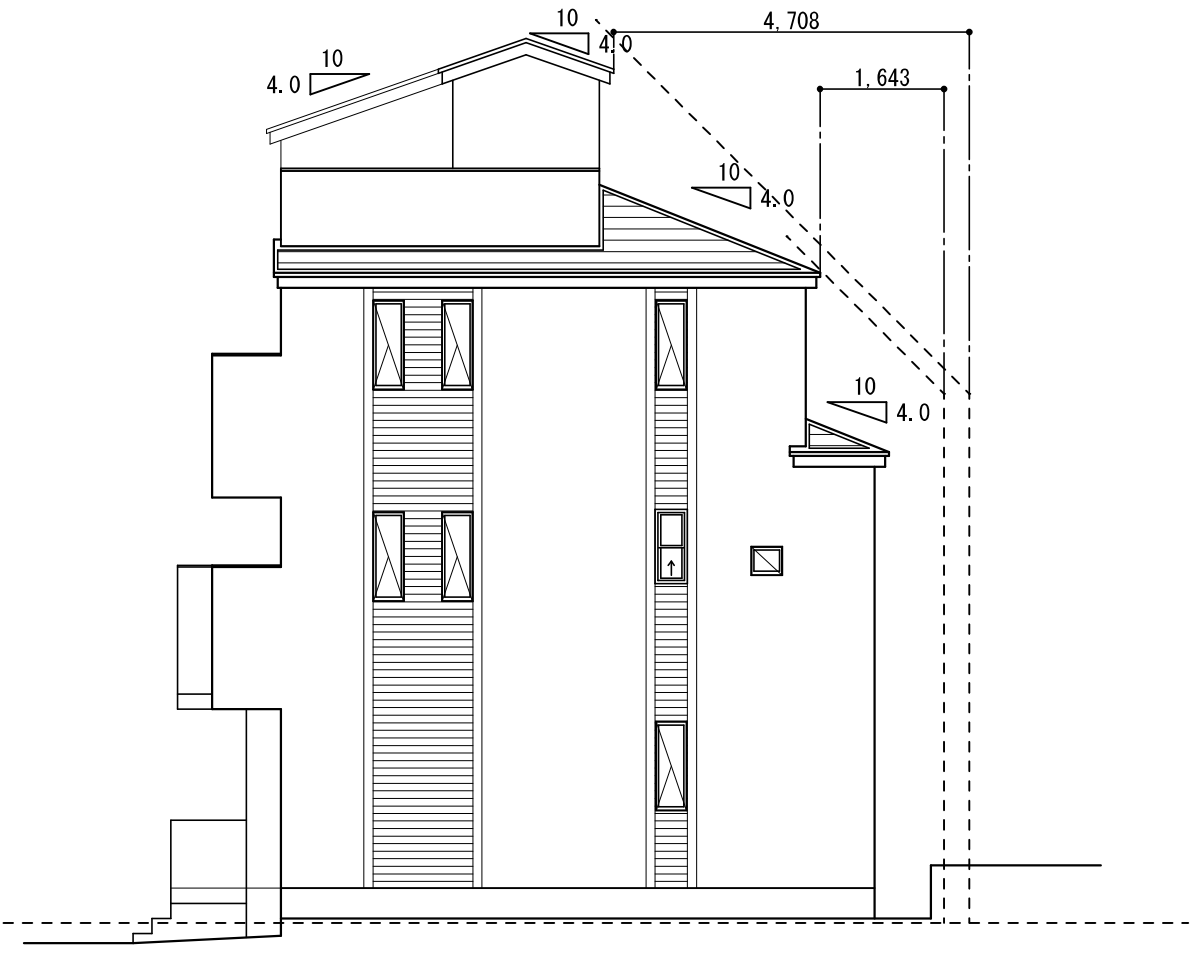
東立面图
