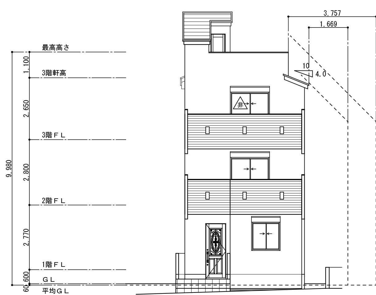
南立面图
