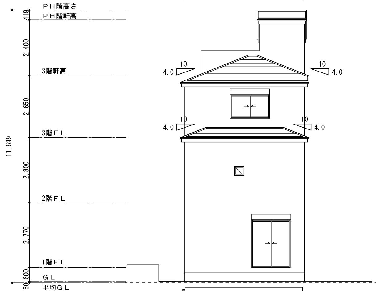
北立面图
