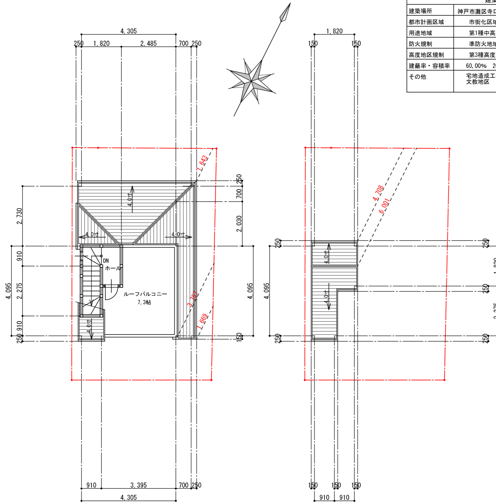
PH階平面図 PH階床面積 : 4.55㎡
